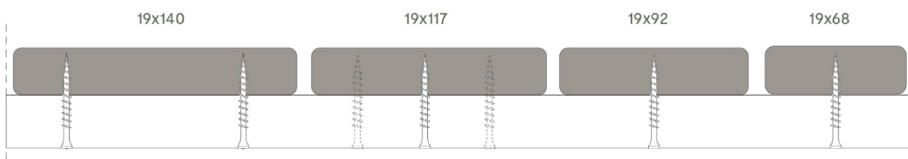
Pav. 3: Dailylenčių tvirtinimas, ruošiant skydus
