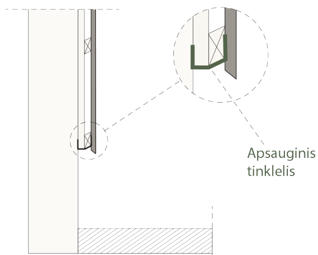
Pav. 2: Apsauginis tinklis montuojant dailylentes vertikaliai ant dvigubo karkaso
