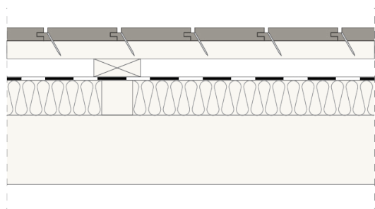
Termomedienos dailylentės Rūta 19x117, prikaltos vinutėmis be galvūčių ant dvigubo medinio karkaso
