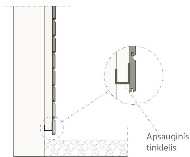
Pav. 3: Apsauginis tinklis montuojant dailylentes Horizontaliai ant viengubo karkaso
