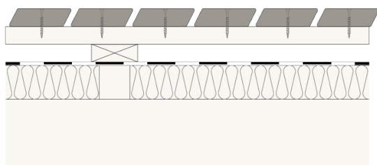
Termomedienos dailylentės Rombas 26x92, prisuktos medšraigčiais ant dvigubo medinio karkaso
